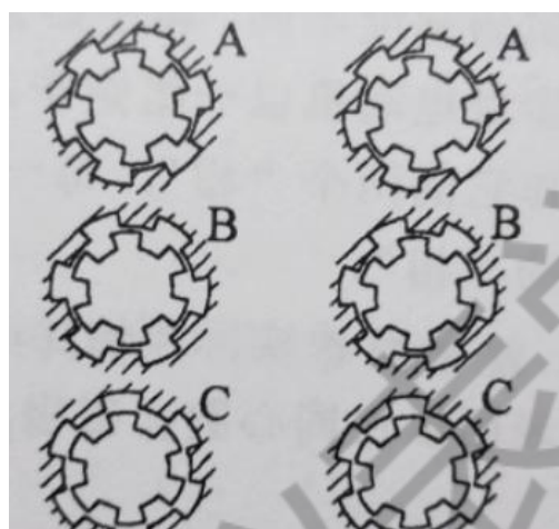
图 2 步进电机的转子和定子示意图
